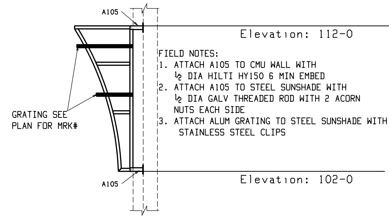
TYP DETAIL 1E18
